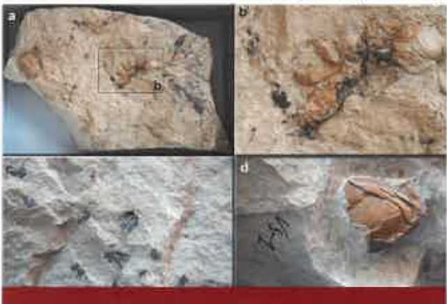
NIDO FÓSIL BARDENAS
